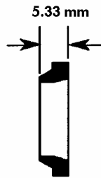
Joint du segment racleur (8012776) Qté: 1
